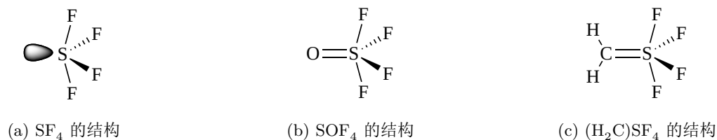
图 11: SF 4 及其衍生物的结构
