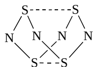
图 13: S_4N_4 的立体结构
